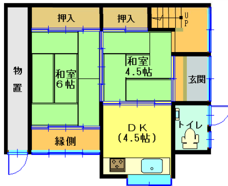
【1階間取図】
