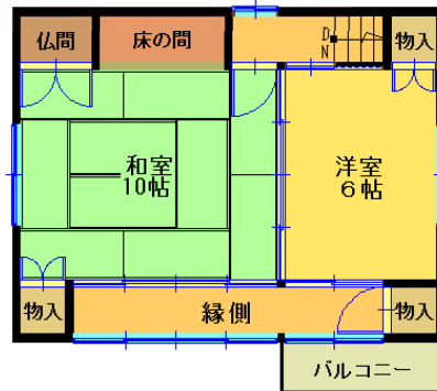
【2階間取図】
