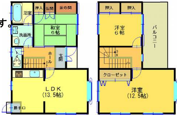
【1階間取図】
